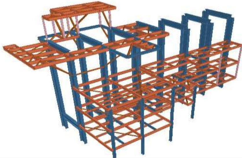
HRSG – Boiler Tekla Model
