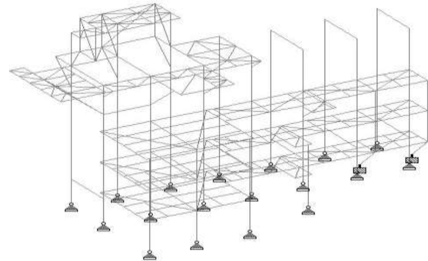
HRSG – Steel STADD Analysis
